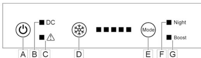
Bild 189: Manöverenhet kylskåp med 12 V kompressor
