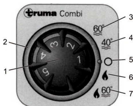
Bild 120: Manöverenhet (TRUMA) för värmeaggregat och varmvattenberedning
