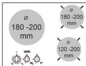
Fig. 202 : Plaques de cuisson
