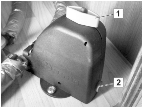
Fig. 104 : Vanne de vidange de sécurité ouverte
