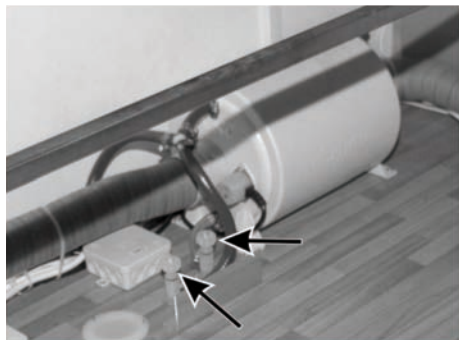
Fig. 94: Chauffe-eau TRUMA et vannes de vidange d'eau
